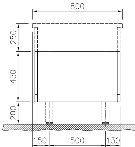
Boven aanzicht
